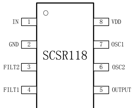
SOP8封装
