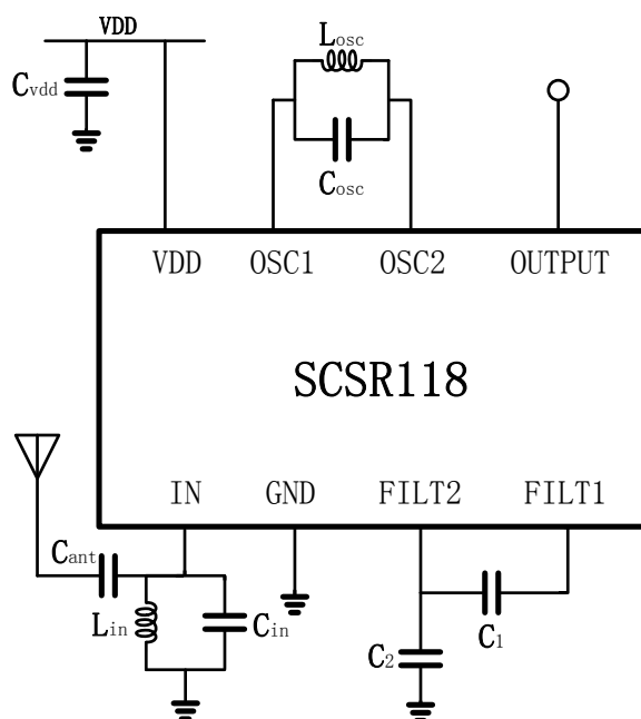
图1. 典型应用电路（一）
