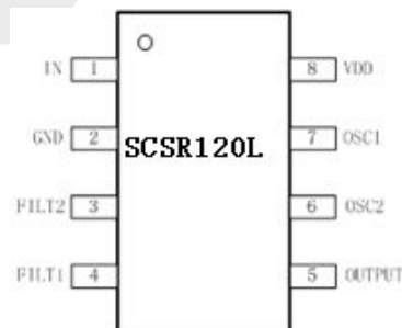
SOP8 Package
